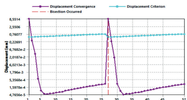
Figura 7. Desplazamiento frenado normal.
