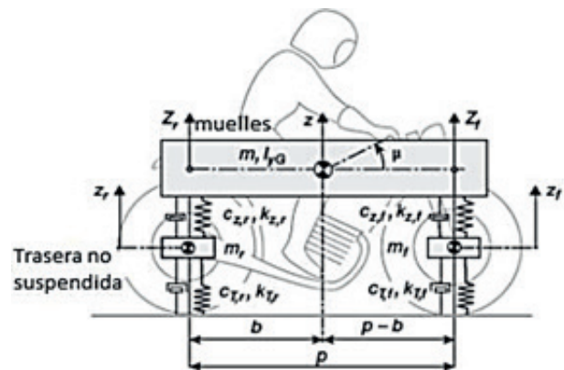
Figura 1. Modelo motocicleta con cuatro grados de libertad
