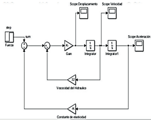
Figura 16. Modelado matemático en simulink
