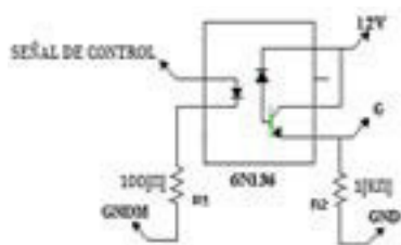
Figura 3. Opto-acoplador 6N136
