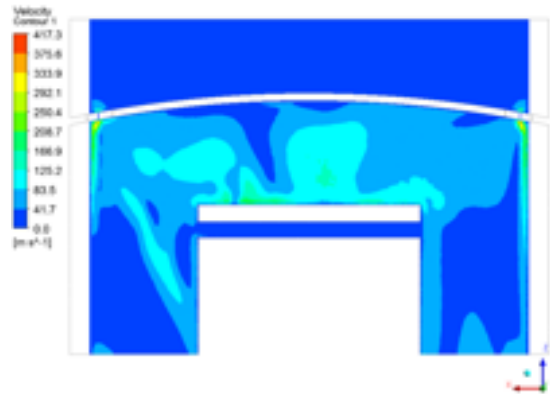
Figura 13. Velocidad de flujo de aire – Persiana 2 a 60km/h
