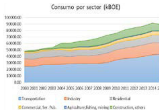
Figura 4. Evolución consumo de energía secundaria
