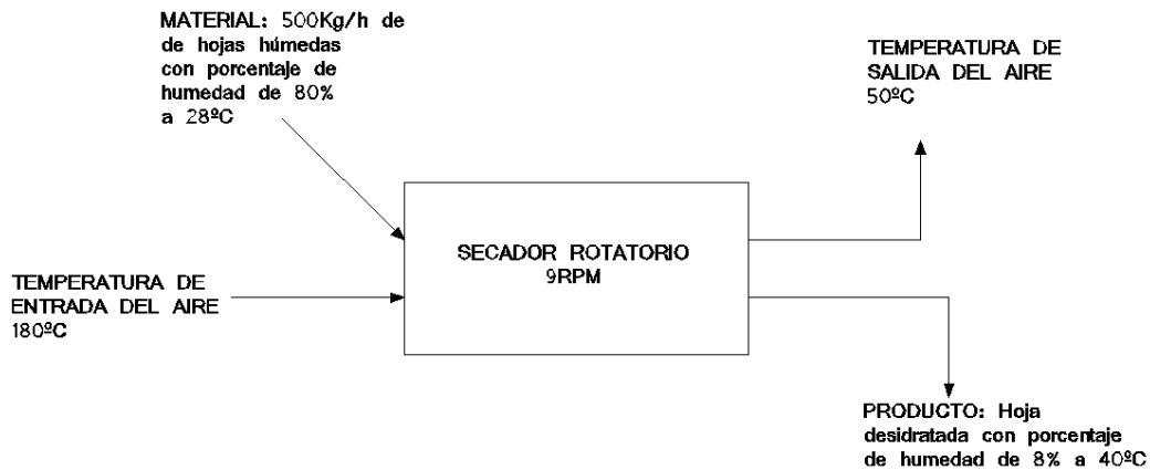
Figura 3.1 Parámetros a utilizar en la máquina
