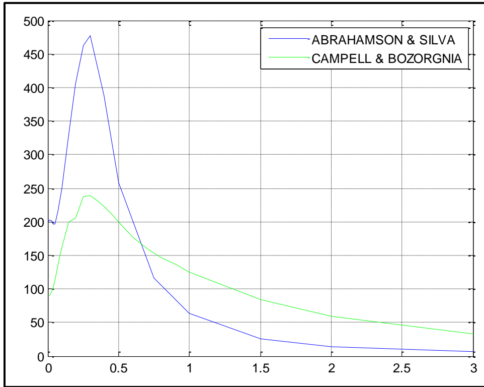
Figura 1.27: Espectro de Diseño de la Falla Real
