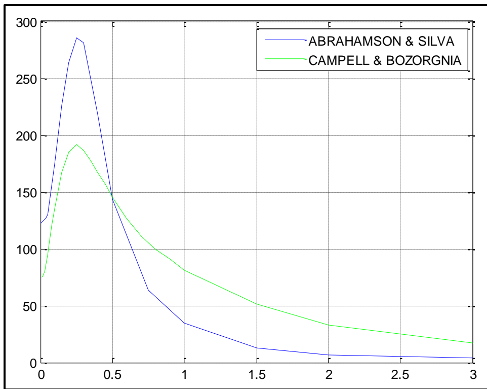
Figura 1.16: Espectro de Diseño de la Falla Domito Norte
