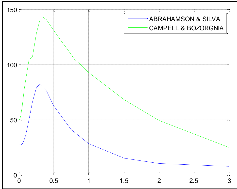
Figura 1.21: Espectro de Diseño de la Falla Prisma
