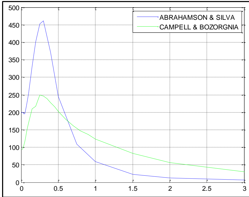
Figura 1.17: Espectro de Diseño de la Falla Engabao
