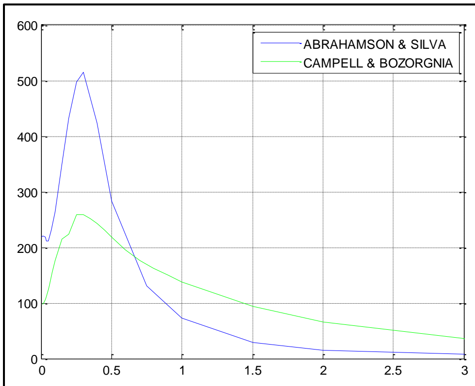
Figura 1.22: Espectro de Diseño de la Falla Santo Tomas
