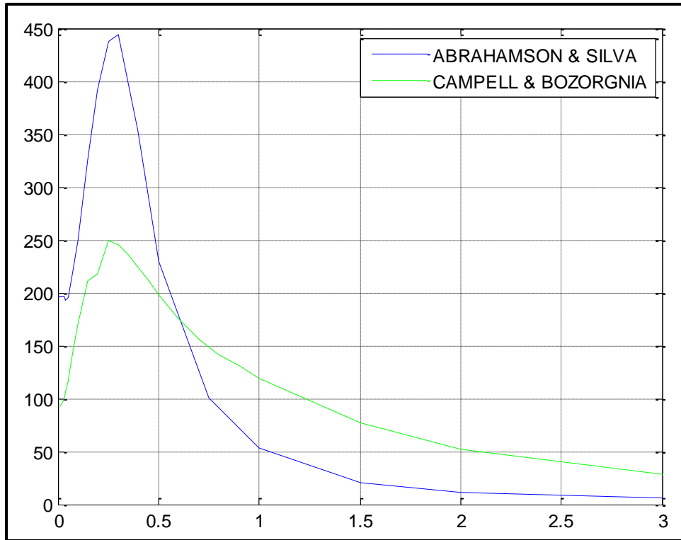
Figura 1.15: Espectro de Diseño de la Falla Data
