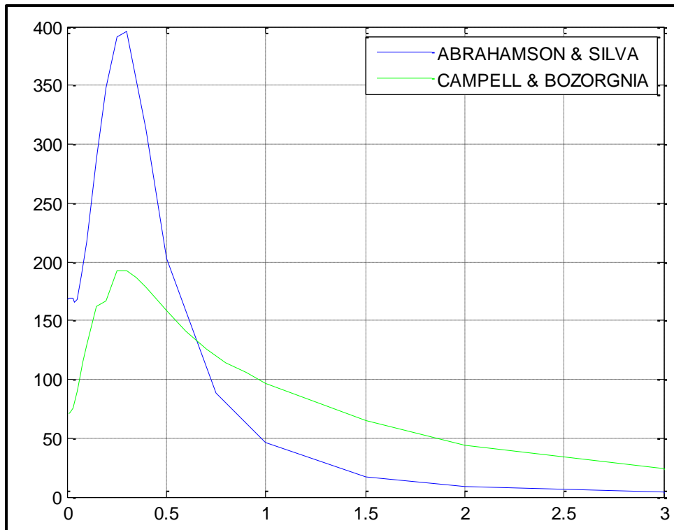
Figura 1.18: Espectro de Diseño de la Falla Jambeli Norte
