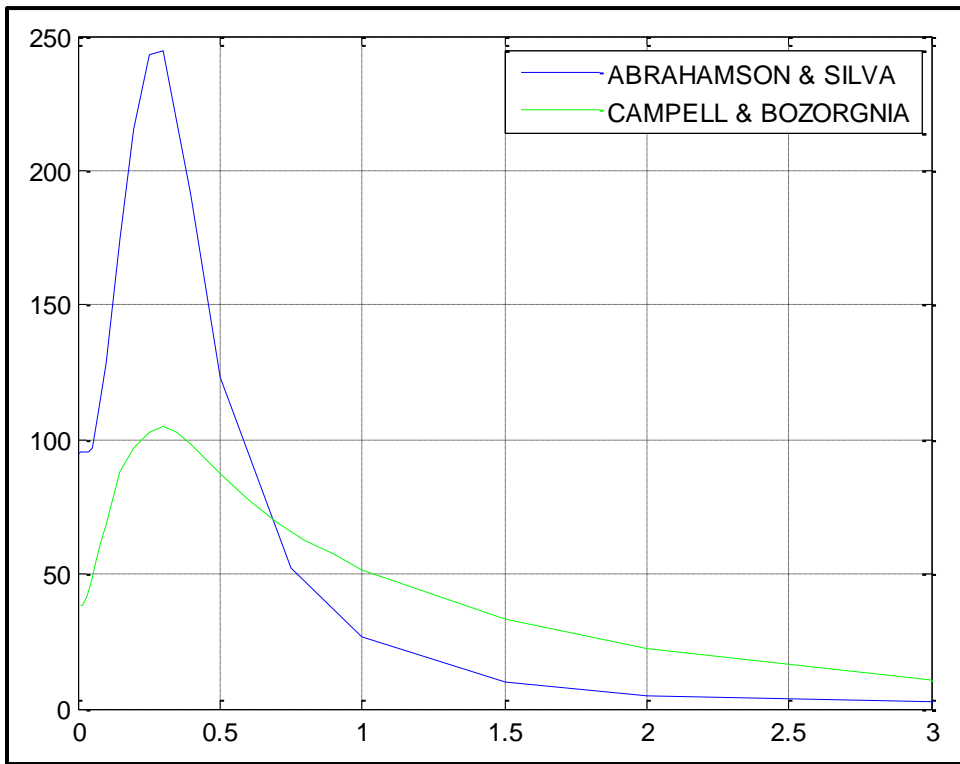
Figura 1.12: Espectro de Diseño de la Falla Catanas
