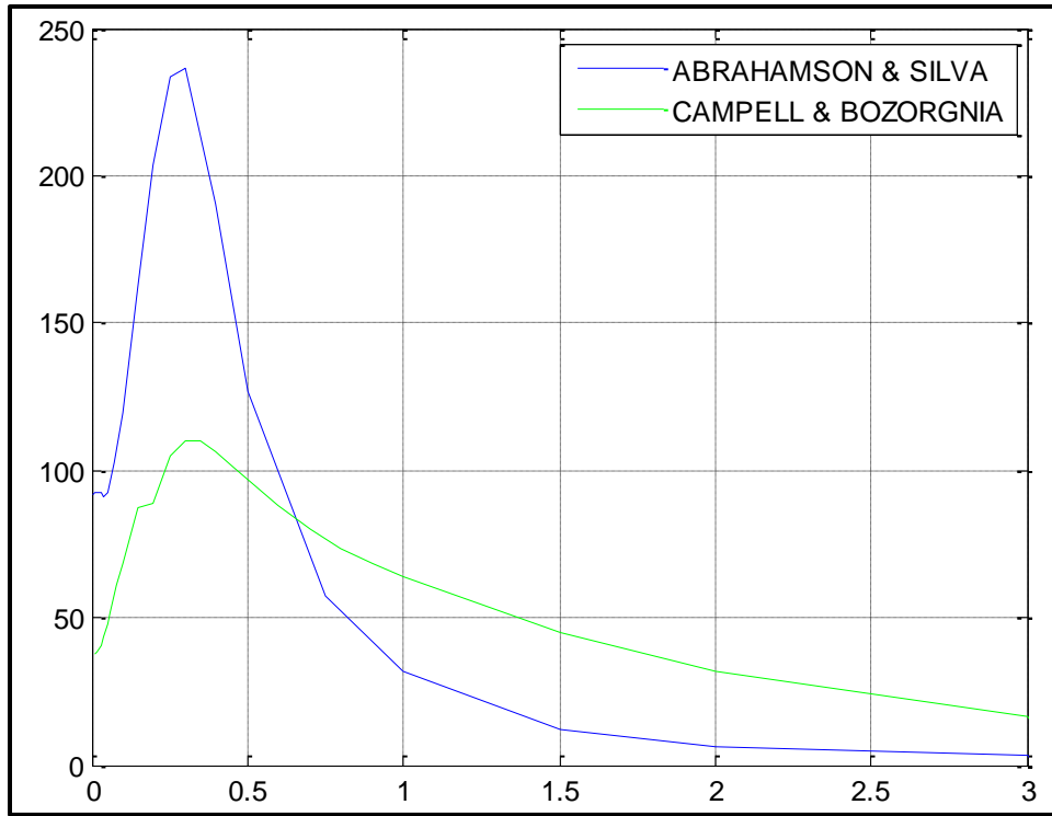
Figura 1.11: Espectro de Diseño de la Falla Carrizal
