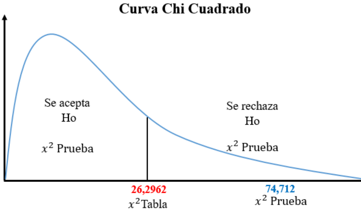
Figura 2. Curva Chi cuadrado, Ayala y Almeida, 2020.
