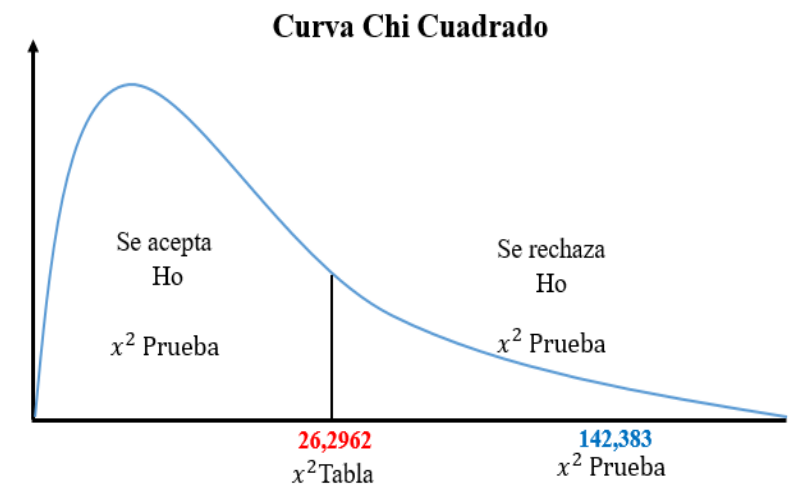
Figura 5. Curva Chi cuadrado, Ayala y Almeida, 2020.
