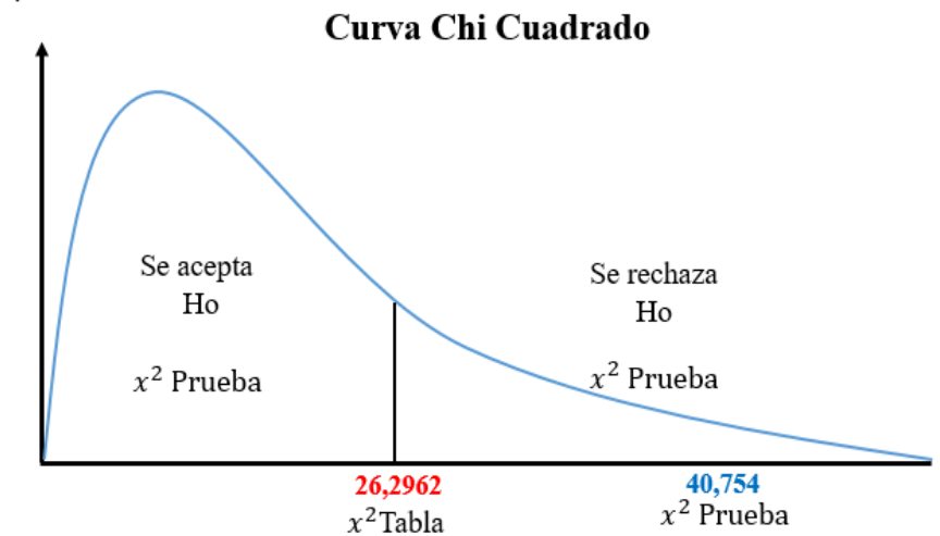
Figura 4. Curva Chi cuadrado, Ayala y Almeida, 2020.
