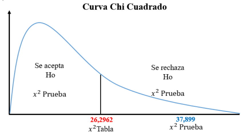
Figura 3. Curva Chi cuadrado, Ayala y Almeida, 2020.
