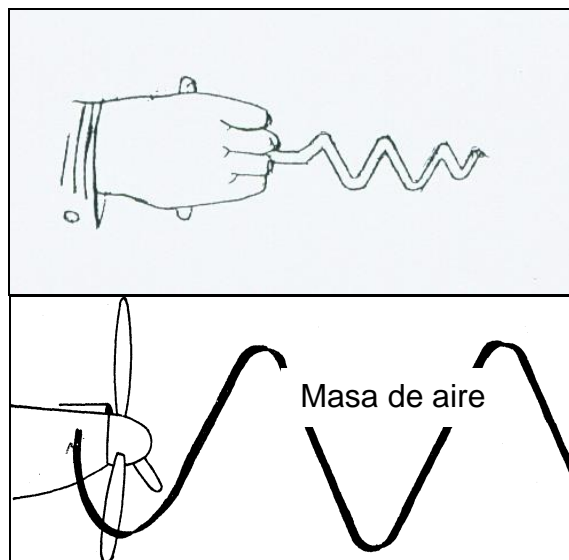
Figura 1.3. Principio de una Hélice
