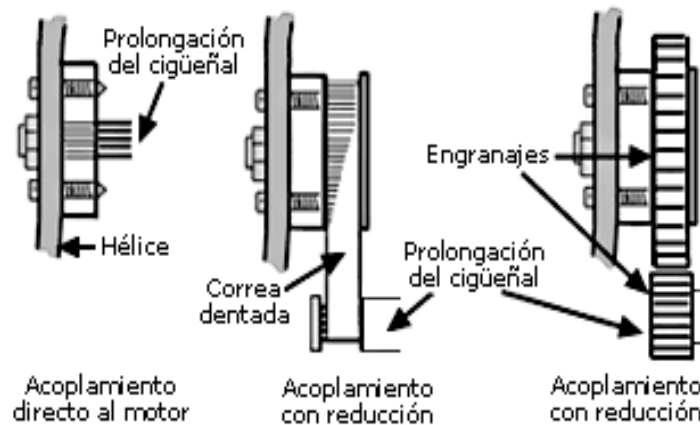
Figura 1.15. Engranajes reductores de velocidad
