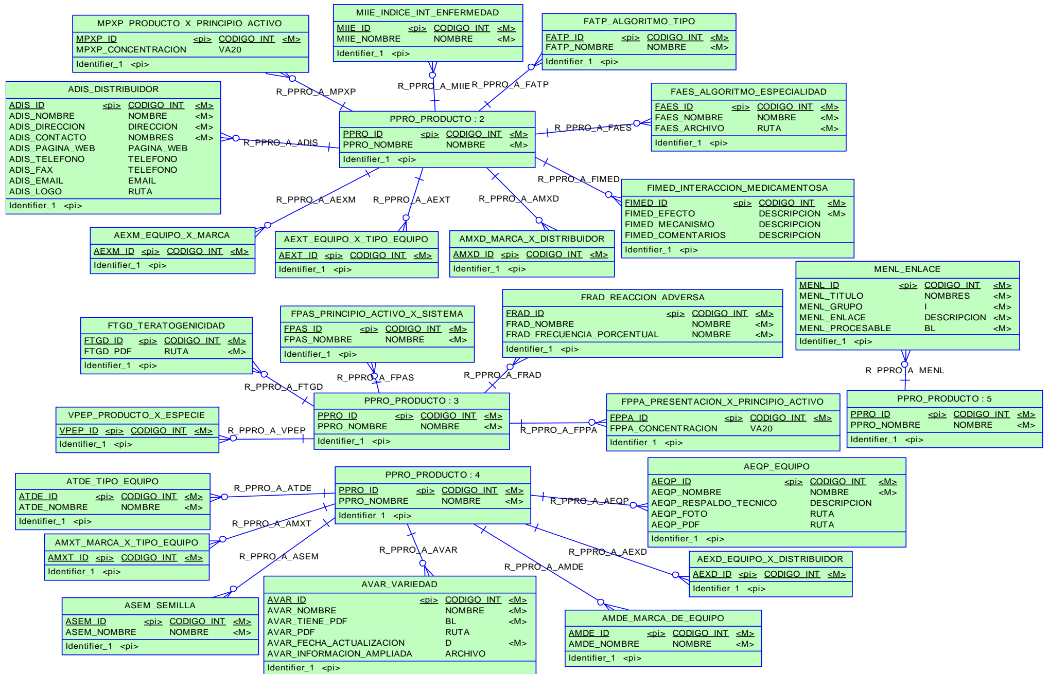
Ilustración 3.77: Diagrama lógico de B.D. "Multiuso - Entidades utilizadas por múltiples Vademecums"
