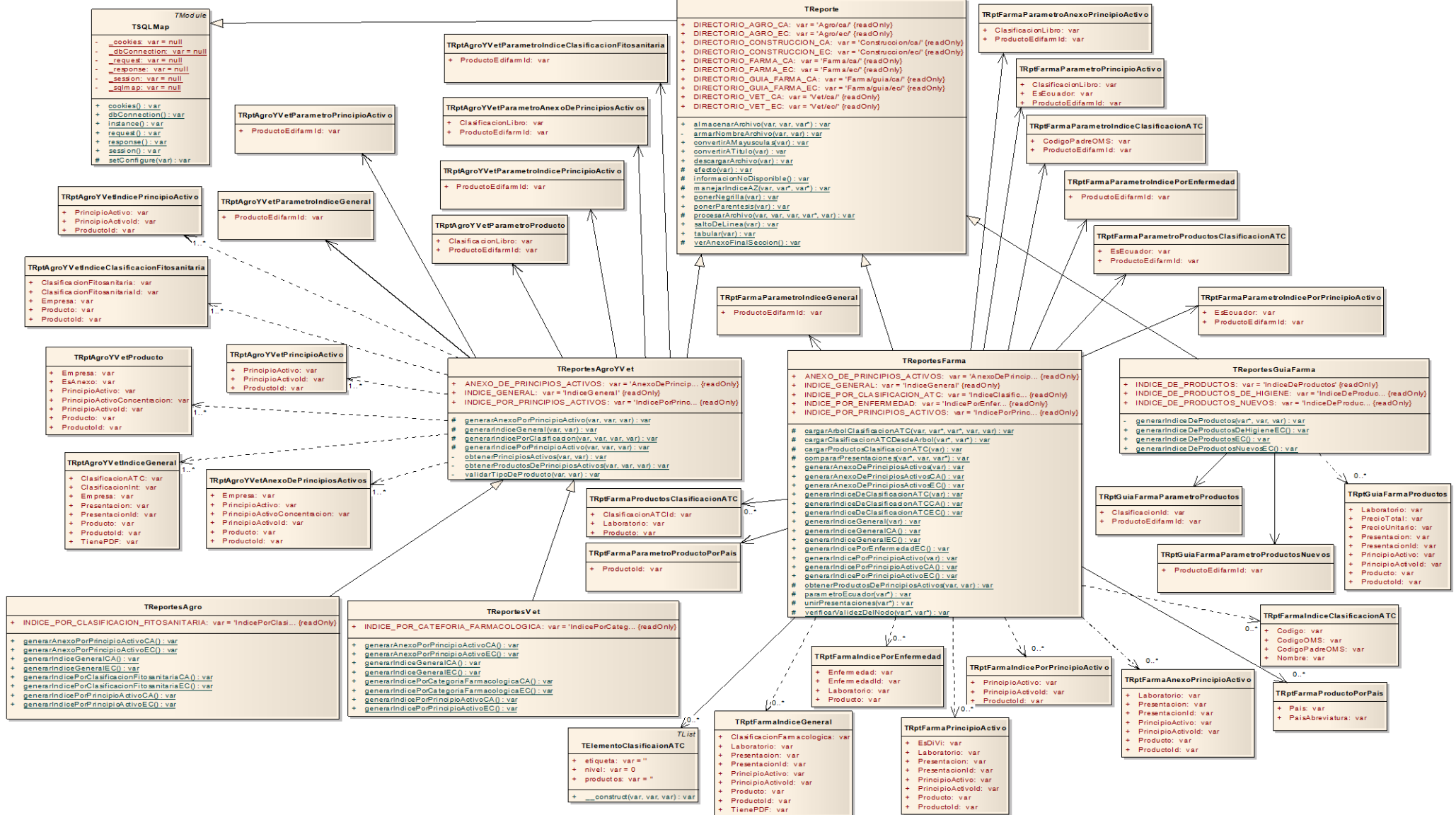
Ilustración 3.68: Diagrama de clases “Clases de Negocio y Persistencia para la Generación de Reportes”
