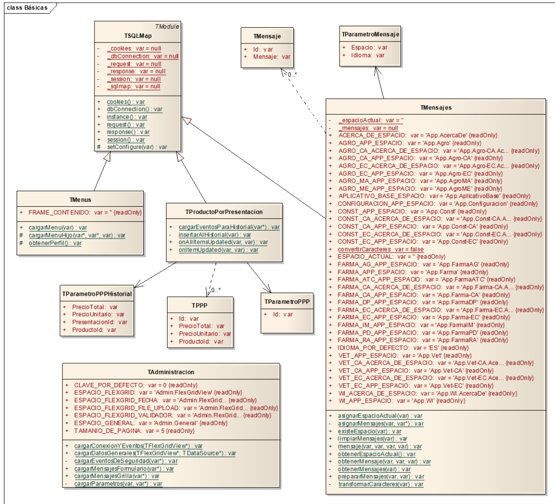
Ilustración 3.59: Diagrama de clases “Clases Básicas del Sistema”
