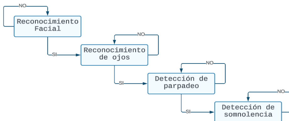
Fig. 1: Etapas del sistema.
