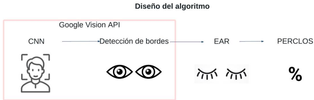
Fig.6: Diseño del Algoritmo
