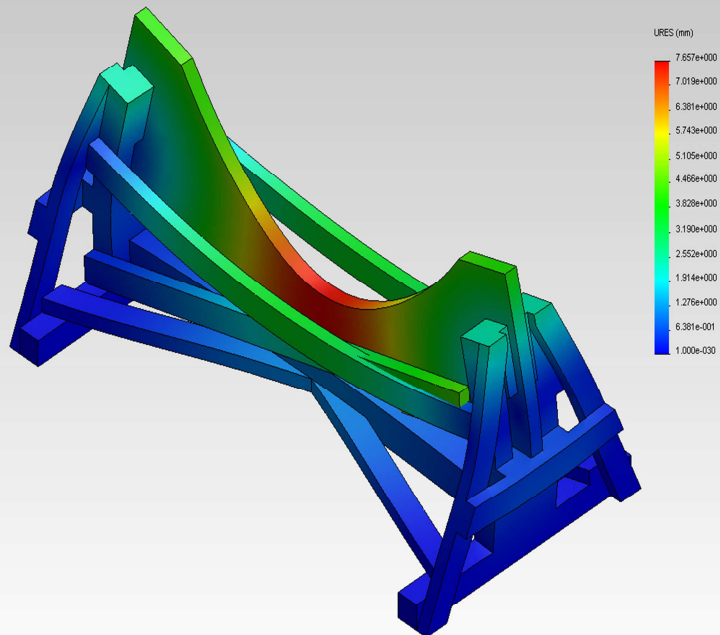
Fig. 3.6 Soporte.Fuselaje Avion Fairchild FH 227 Estudio 1-Desplazamientos-Desplazamientos1
