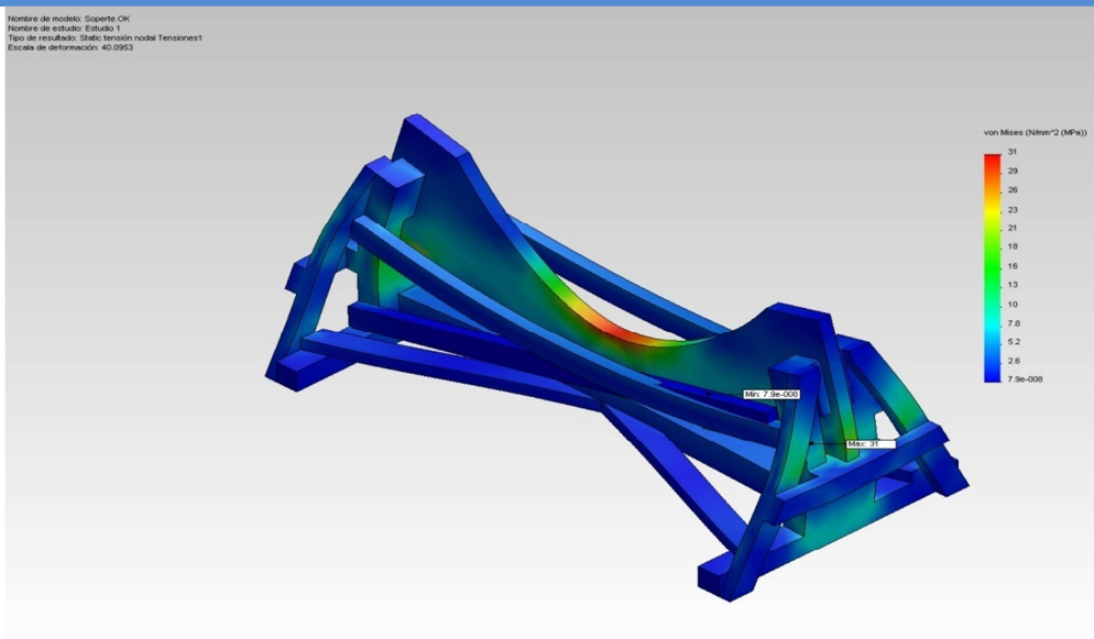
Fig. 3.5 Soporte.Fuselaje Avion Fairchild FH 227
