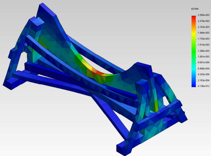
Fig. 3.7 Soporte.Fuselaje Avion Fairchild FH 227 1-Deformaciones unitarias-Deformaciones unitarias1
