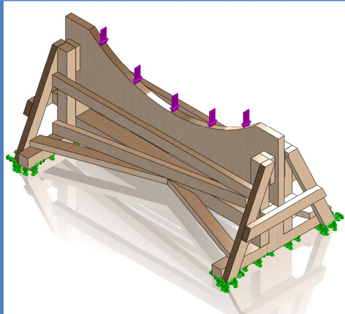
Fig. 3.3 Nombre del modelo: Soperte.Fuselaje Avion Fairchild FH 227 Configuración actual: Predeterminado
