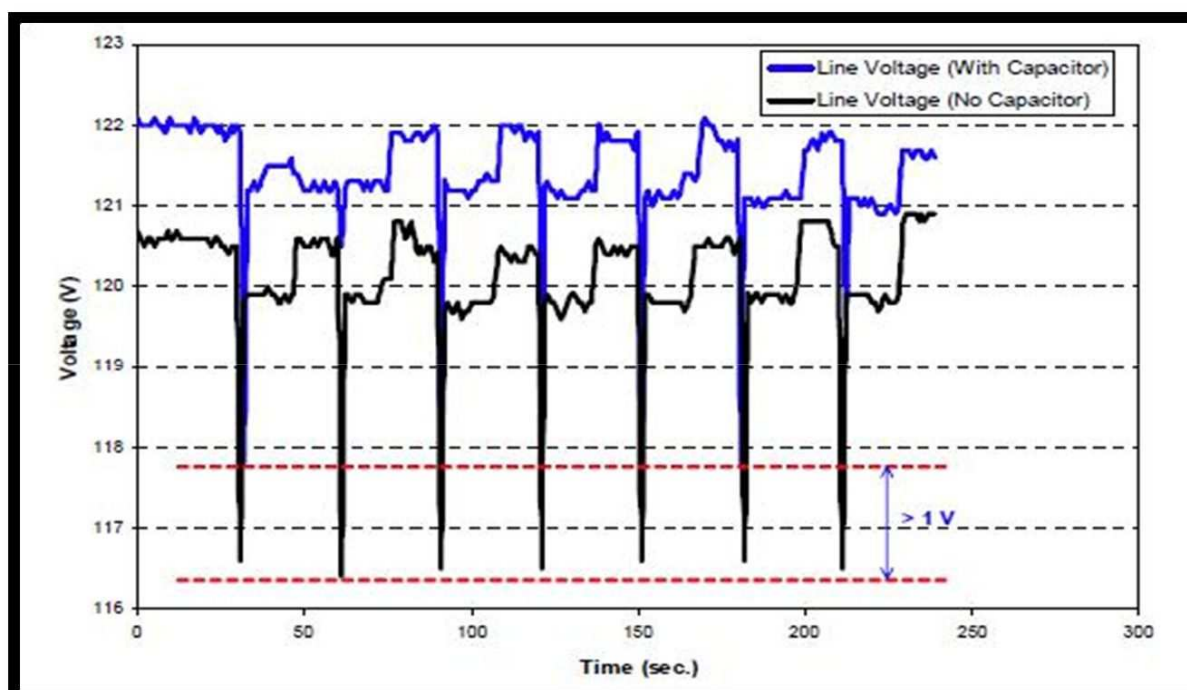
Figura 2.4: EFECTO DE LAS VARIACIONES DE VOLTAJE
