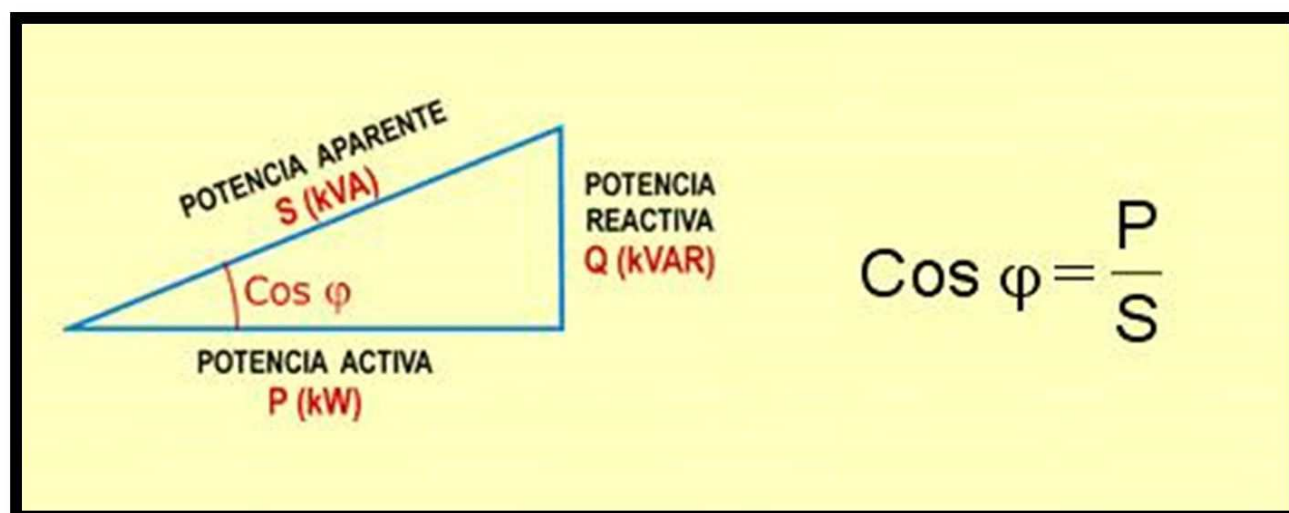
Figura 2.5: TRIANGULO DE POTENCIA Fuente: ramaucsa.wordpress.com
