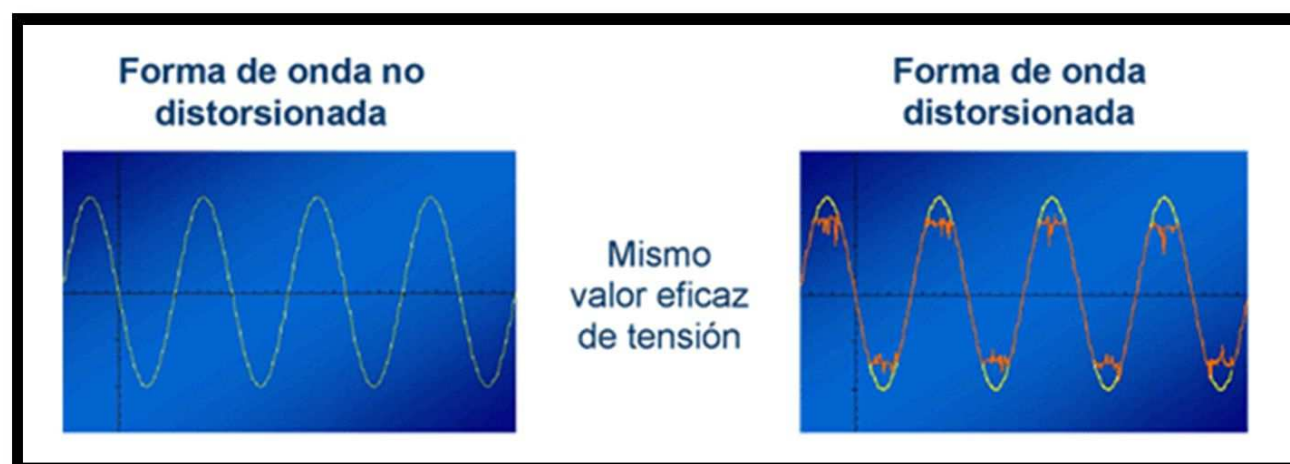
Figura 2.6: DISTORSIÓN ARMÓNICA Fuente: www.prolyt.com
