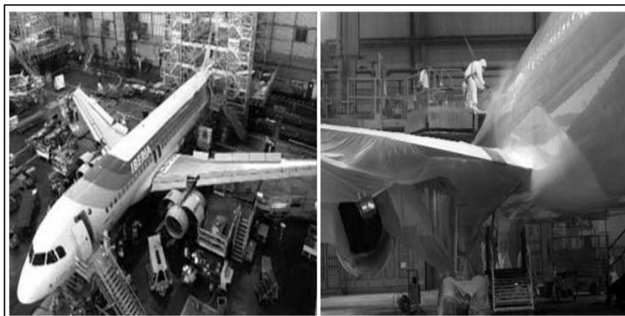
Figura 9 Mantenimiento mayor
