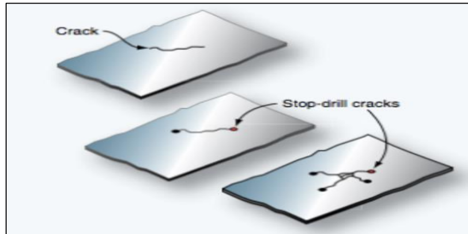
Figura 10 Reparación estructural
