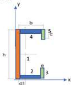
Figura 3. Centroide
