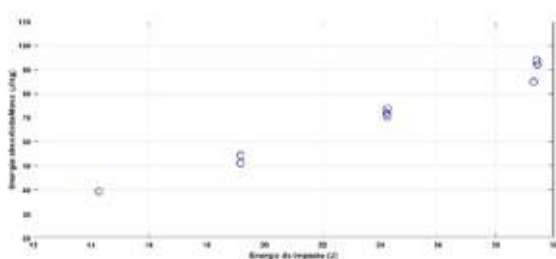
Figura 6. Energía absorbida/masa vs. energía de impacto para la estructura tubular.
