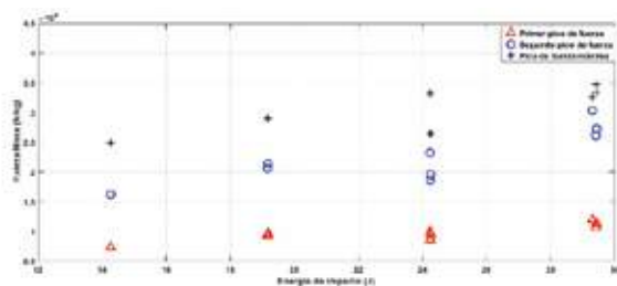
Figura 5. Picos de fuerza/masa vs. energía de impacto para la estructura tubular
