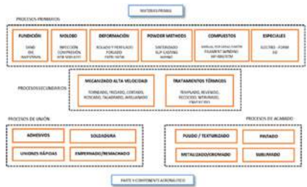
Figura 16. Procesos de Manufactura para componentes aeronáuticos.
