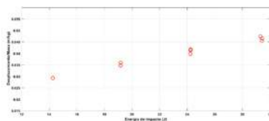
Figura 7. Desplazamiento máximo/masa vs. energía de impacto para la estructura tubular.
