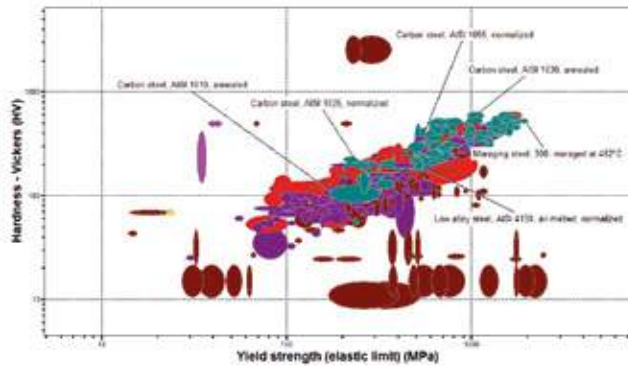
Figura 7. Relación Resistencia vs Dureza de aleaciones de acero utilizado en aeronáutica.
