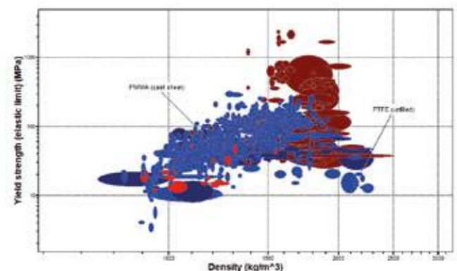
Figura 11. Relación Resistencia vs Densidad plásticos utilizado en aeronáutica
