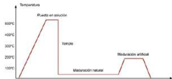
Figura 4. Tratamiento térmico de endurecimiento estructural del aluminio
