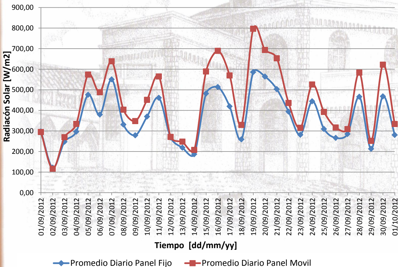
PROMEDIO DIARIO DE RADIACIÓN SOLAR
