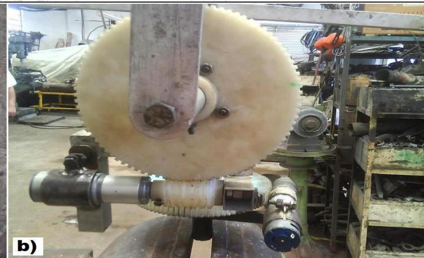
a) Base para motorreductor y eje principal, b) base de sujeción del motorreductor en altura solar.
