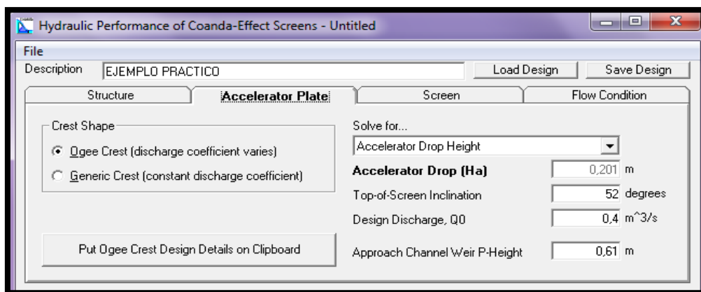
Figura 1.5: Ingreso del caudal de diseño
